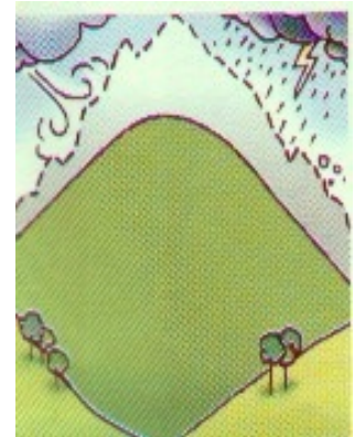
colline strutturali
