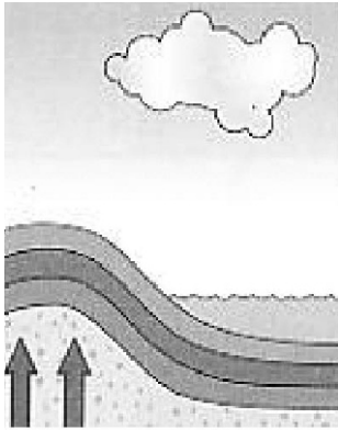
colline tettoniche
