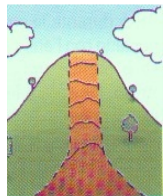
colline vulcaniche
